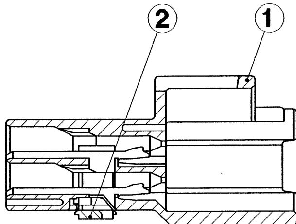
SEC. A-A
