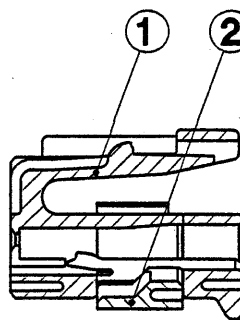
SEC. A-A
