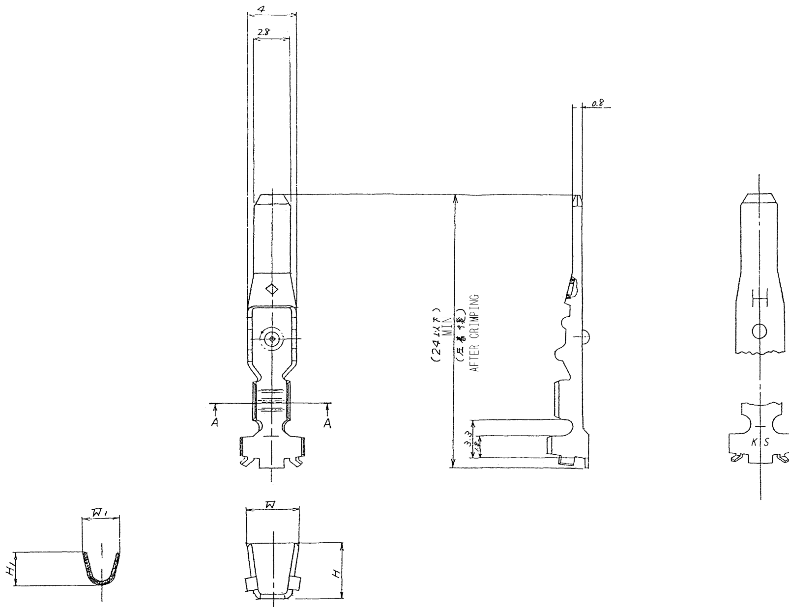
SECTION A-A
