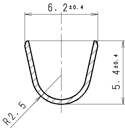
SEC. A-A
