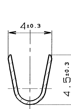
SEC. A-A
