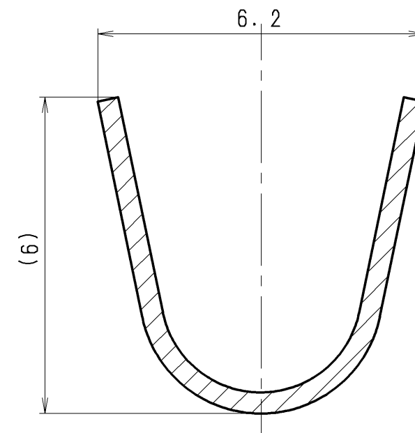
SECTION A-A (10:1)
