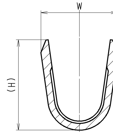
SECTION B-B (10:1)
