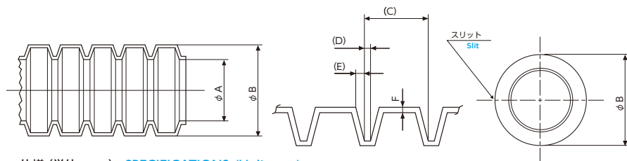
仕様 (単位: mm) SPECIFICATIONS (Unit: mm)
