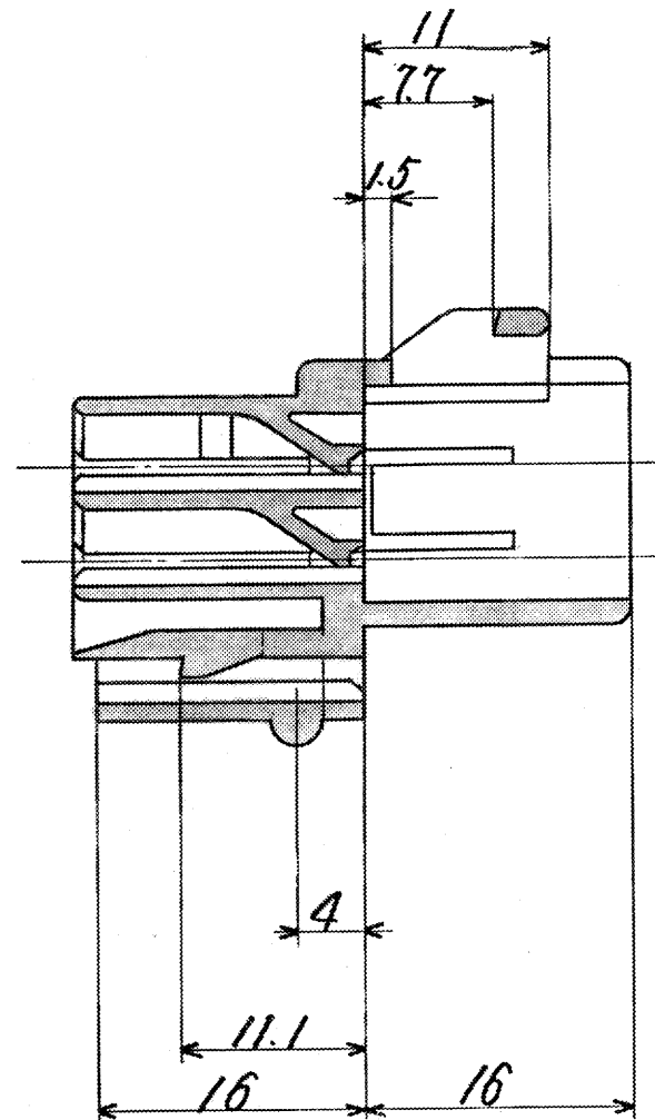
断面 A-A
