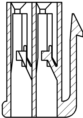
SEC. A-A
