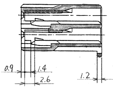
断面 A-A
