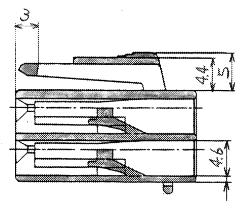
断面 B-B
