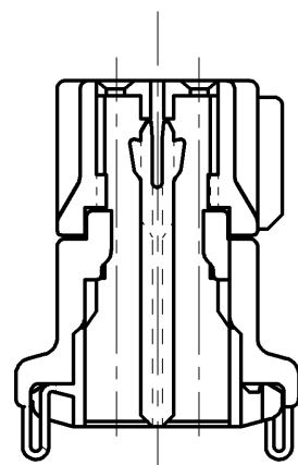
SEC. A-A
