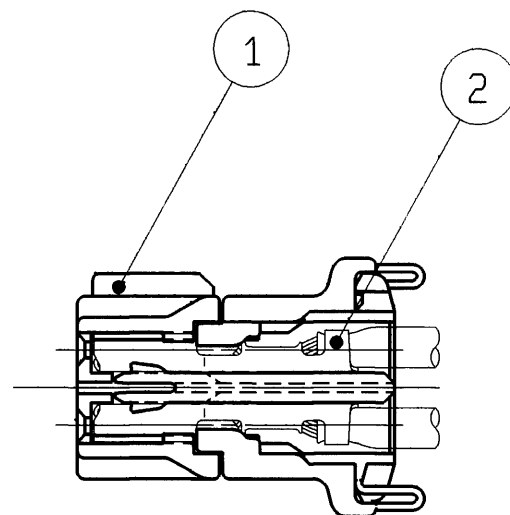
断面 A-A
