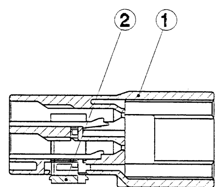
SEC. A-A
