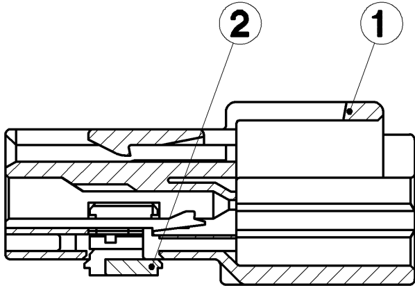
SEC. A-A
