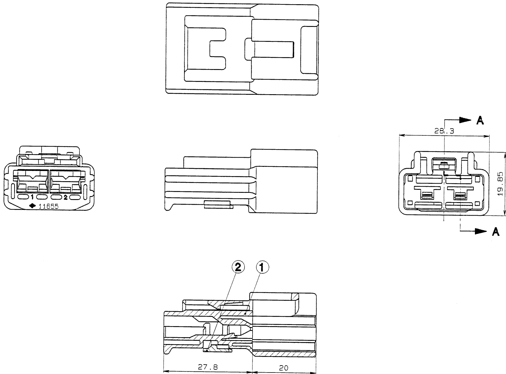
SEC. A-A
