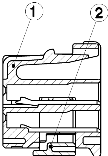
SEC. A- A
