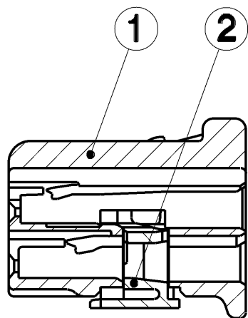
SEC. A-A
