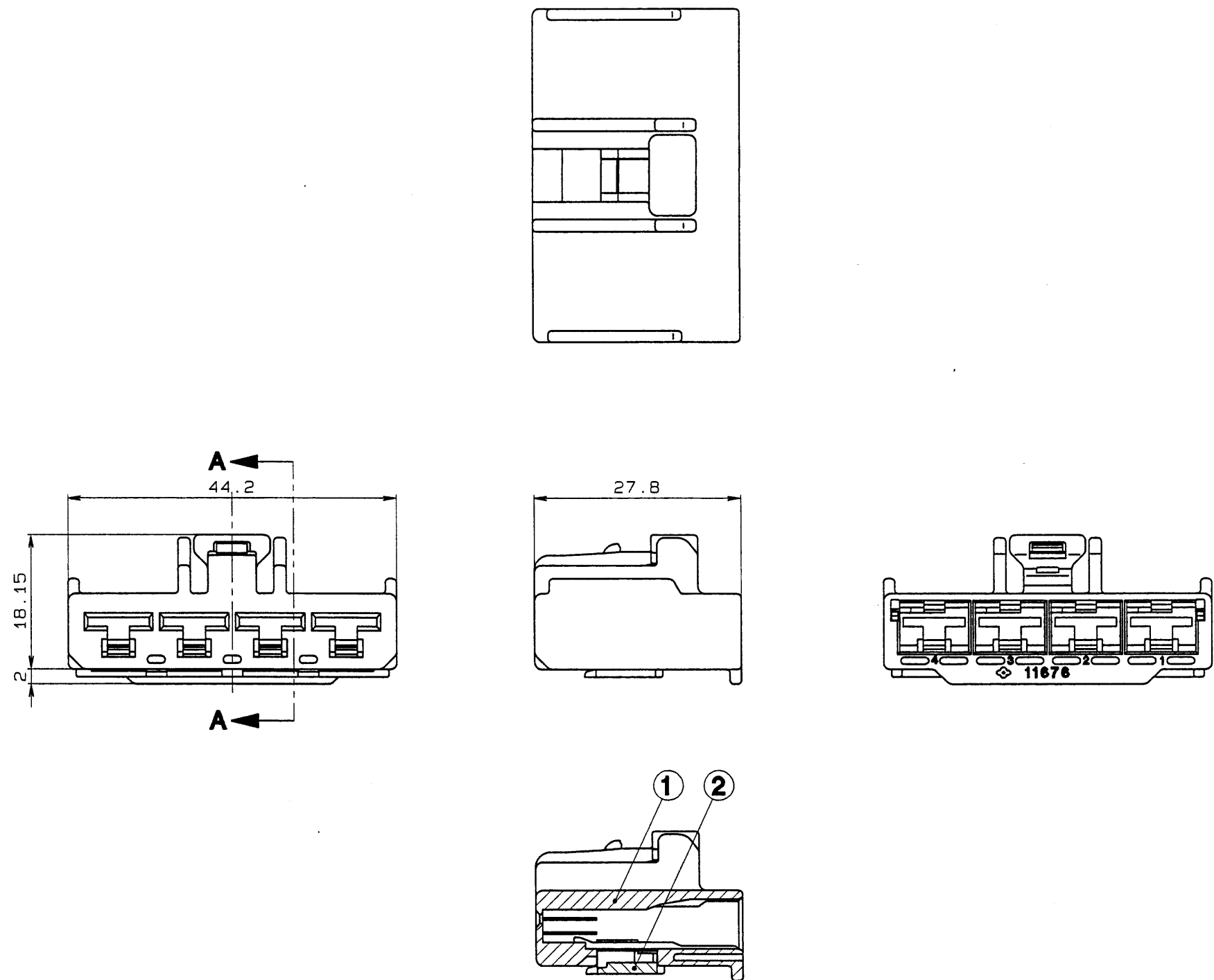
SEC. A-A
