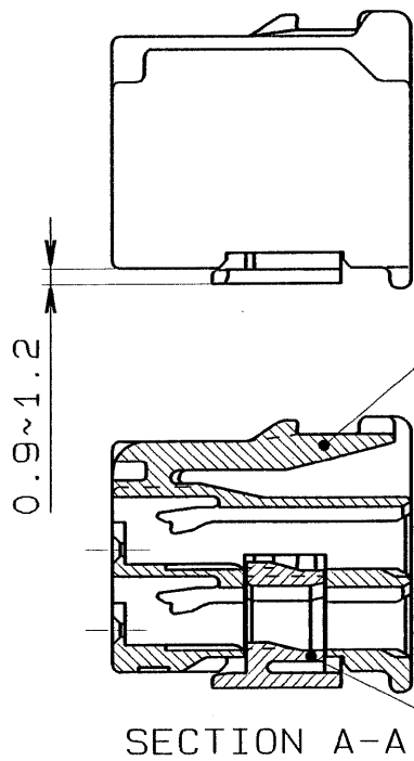
ハウジング ① HOUSING
