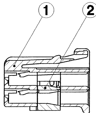
SEC. A-A
