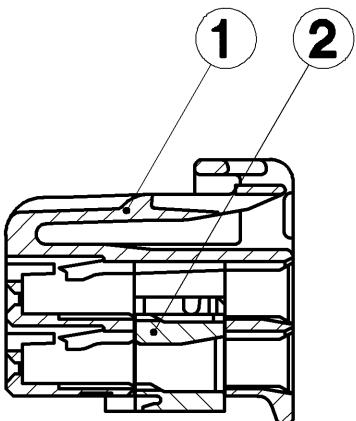
SEC. A-A
