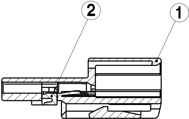
SEC. A- A
