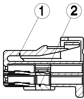
SEC. A-A
