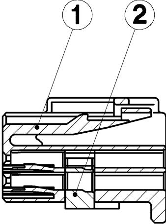
SEC. A-A
