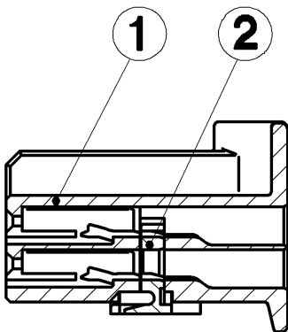
SEC. A-A
