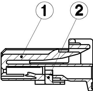
SEC. A-A
