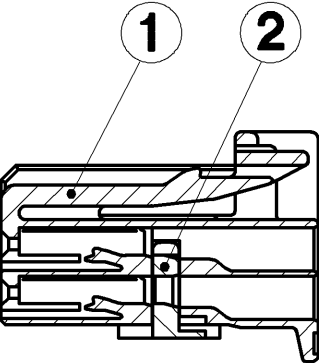
SEC. A-A
