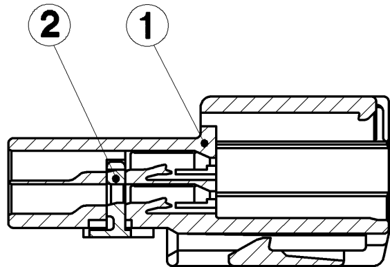
SEC. A-A
