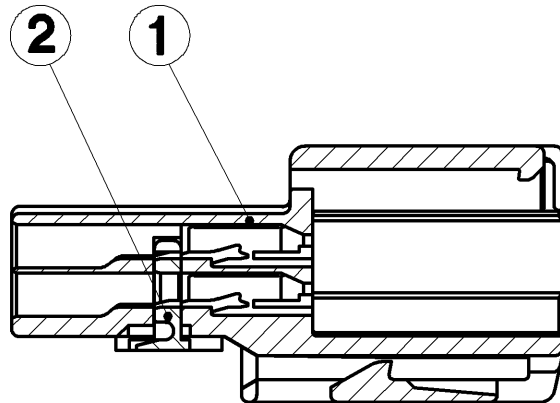
SEC. A-A
