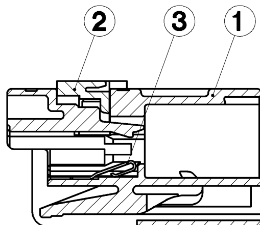
SEC. A-A
