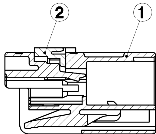
SEC. A-A
