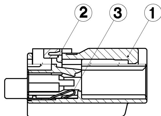
SEC. A-A
