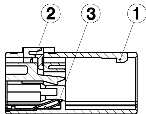
SEC. A-A
