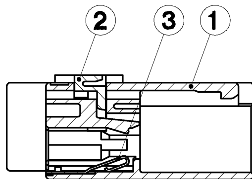
SEC. A-A
