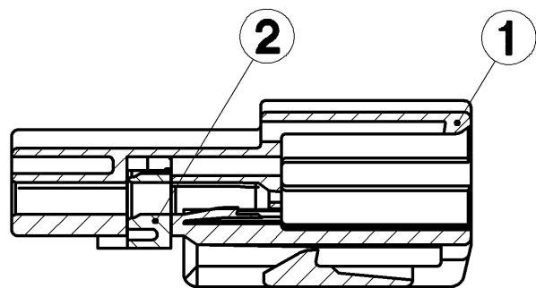
SEC. A-A
