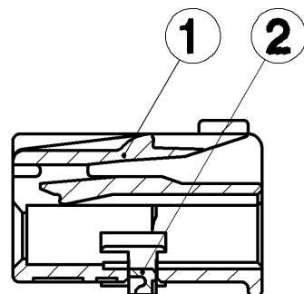
SEC. A-A
