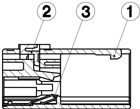
SEC. A-A
