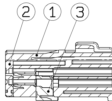
SEC. A-A
