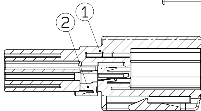
SEC. A-A
