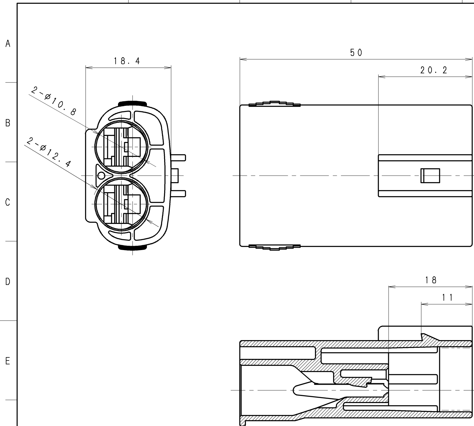
SECTION A-A
