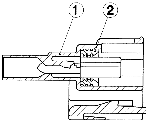
SEC. A-A
