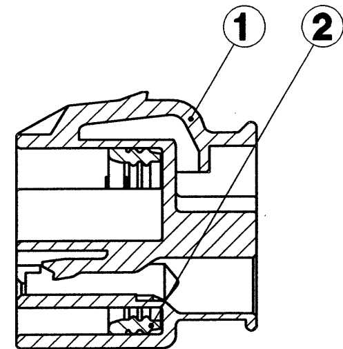
SEC. A-A
