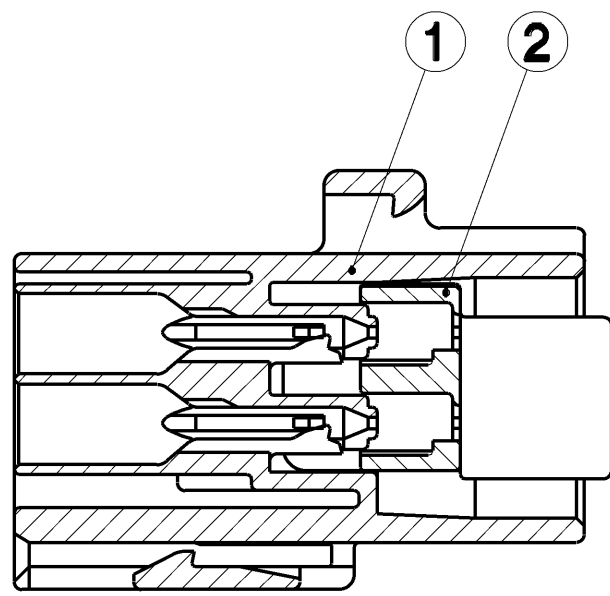
SEC. A-A
