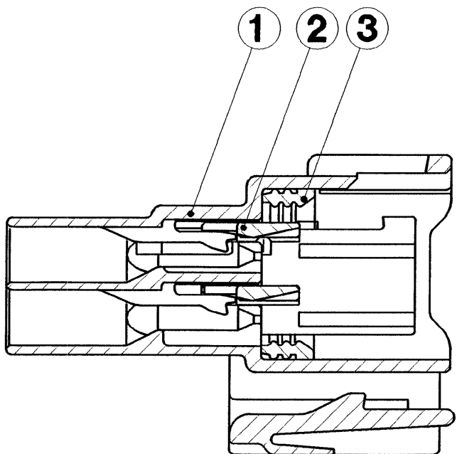
SEC. A-A
