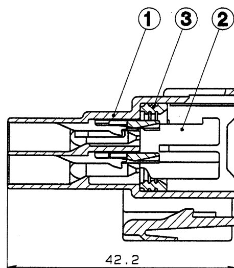
SEC. A-A
