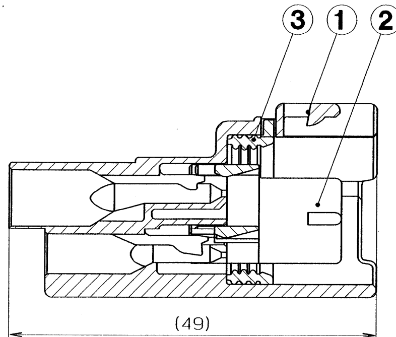
SEC. A-A
