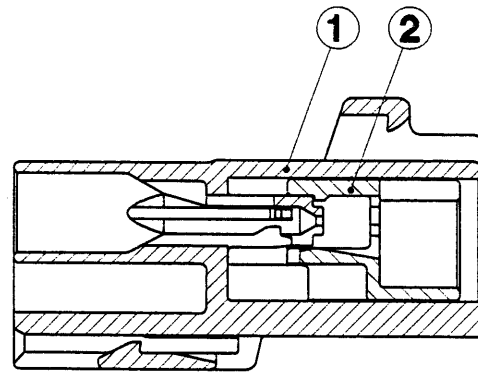
SEC. A-A
