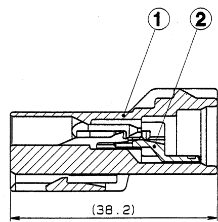
SEC. A-A
