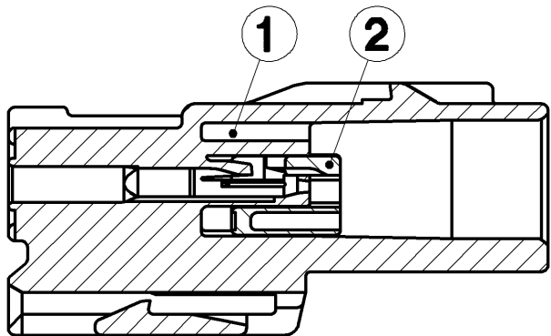
SEC. A-A
