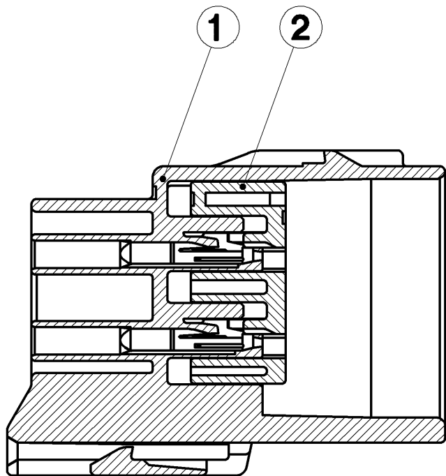
SEC. A-A
